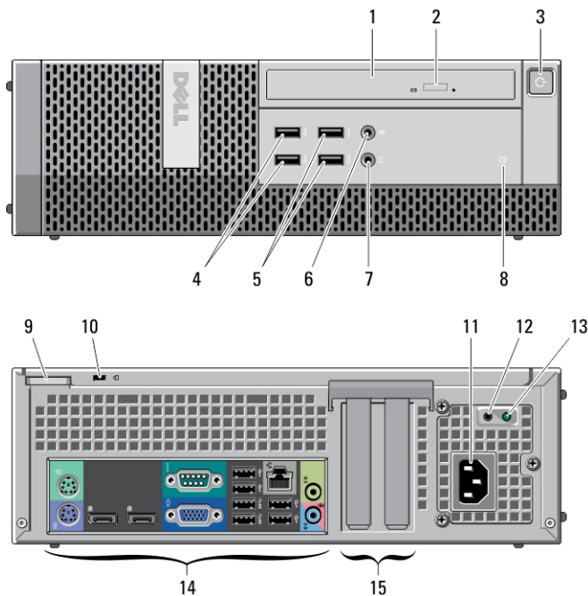
Obrázek 3. Pohled zepředu a zezadu na panel provedení Small Form Factor
